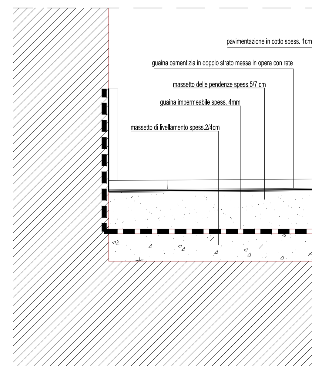
PARTICOLARE SCALA 1:5
