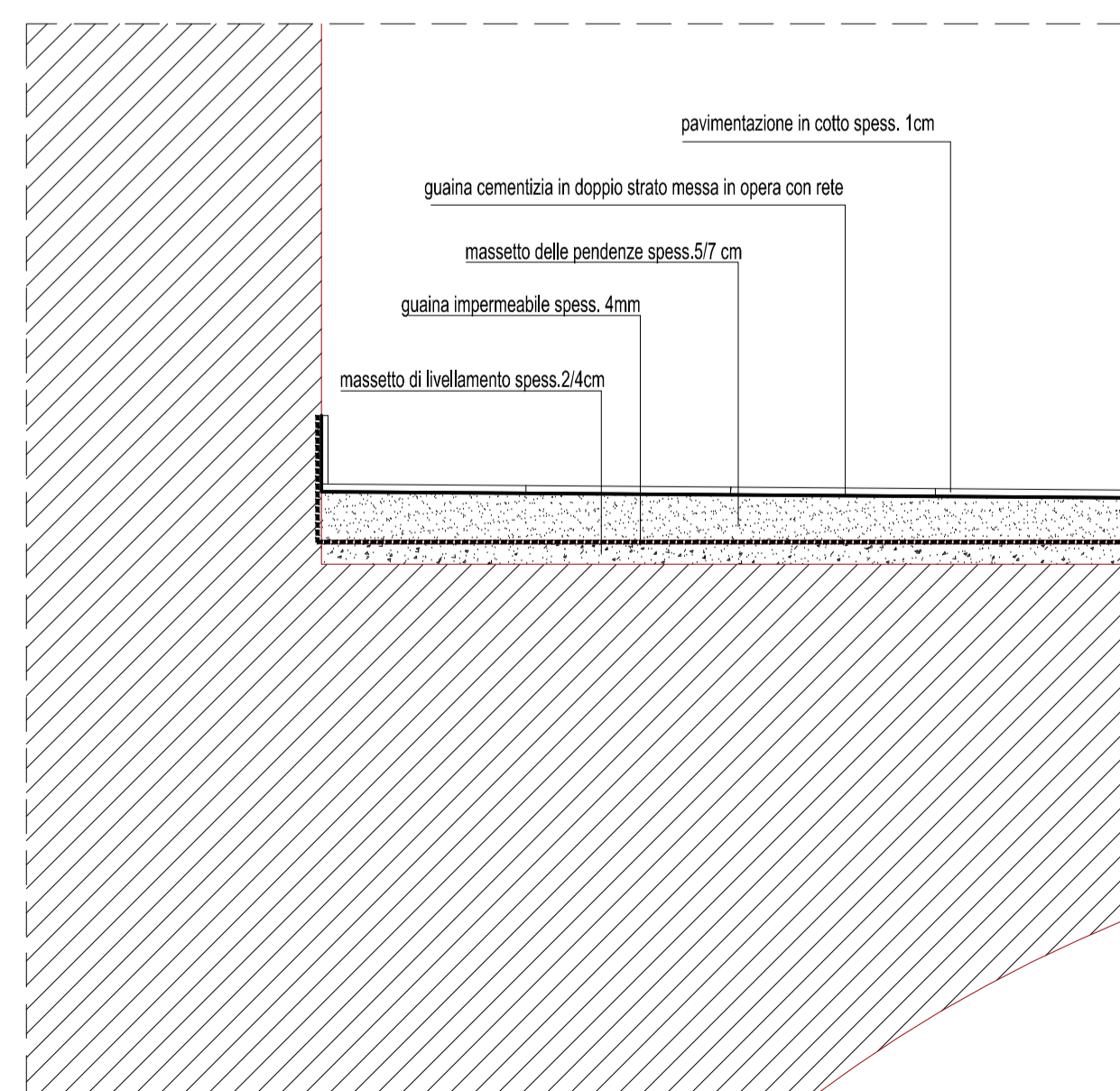
PARTICOLARE SCALA 1:20
