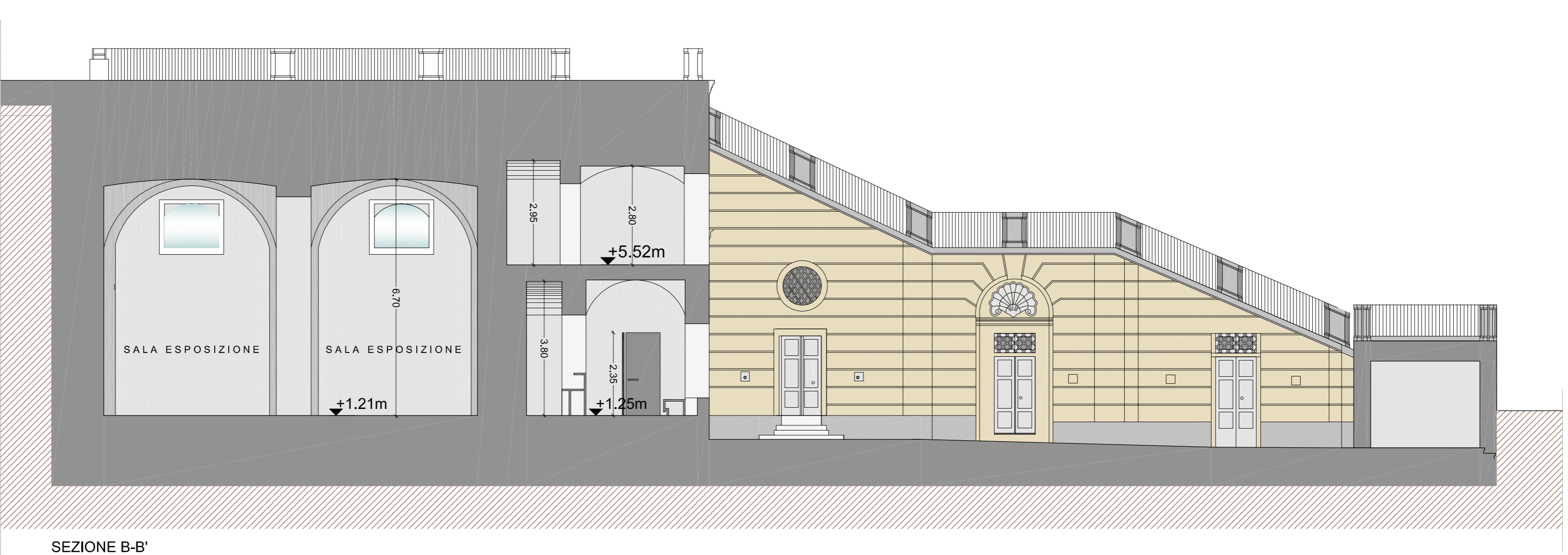
SEZIONE B-B'
